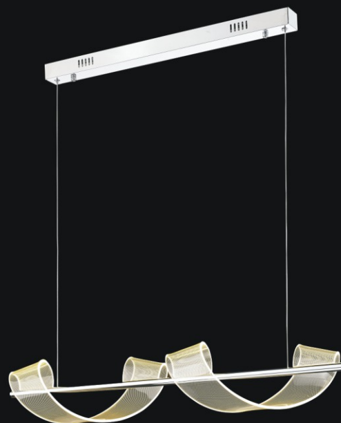
WE452.02.123 L900 W200 H1500 LED, 28W
