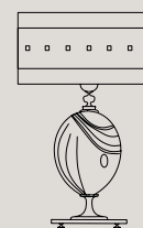
LG1 1 E27 x 60W Ø 40 cm - H 77 cm
