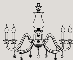
L5 5 E14 x 40W Ø 82 cm - H 80 cm
