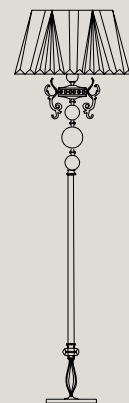
PT1 1 E27 x 60W Ø 45 cm - H 180 cm
