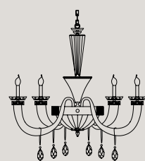
L6 6 E14 x 40W Ø88 cm - H 74 cm
