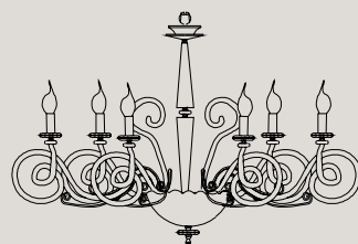
L10 10 E14 x 40W Ø 99 cm - H 85 cm
