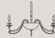
A2 2 E14 x 40W 40x26 cm - H 42 cm
