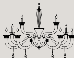
L6+3+3 12 E14 x 40W Ø 110 cm - H 81 cm
