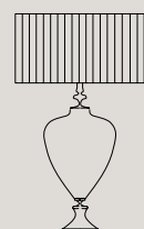
LG1 1 E27 x 60W Ø 40 cm - H 66 cm
