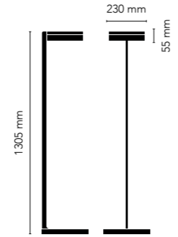
BLADE F1 SLIM 12.5W LED - 220-240V
