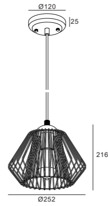
OL040 E27 Cotout :N/A
