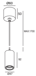
OL039 E27 Cotout :N/A
